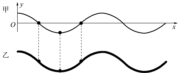
甲: 横波的图像 乙: 绳上的横波
