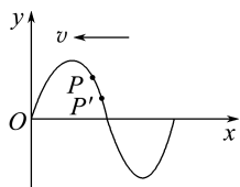
P向下运动
