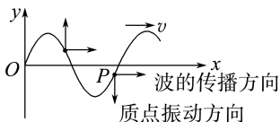
质点振动方向
