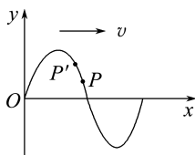
P向上运动
